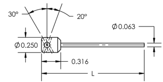
H-20/30 (TUNGSTEN HOLDER ASSEMBLY 20 & 30 DEG P/N: 002-0772)
